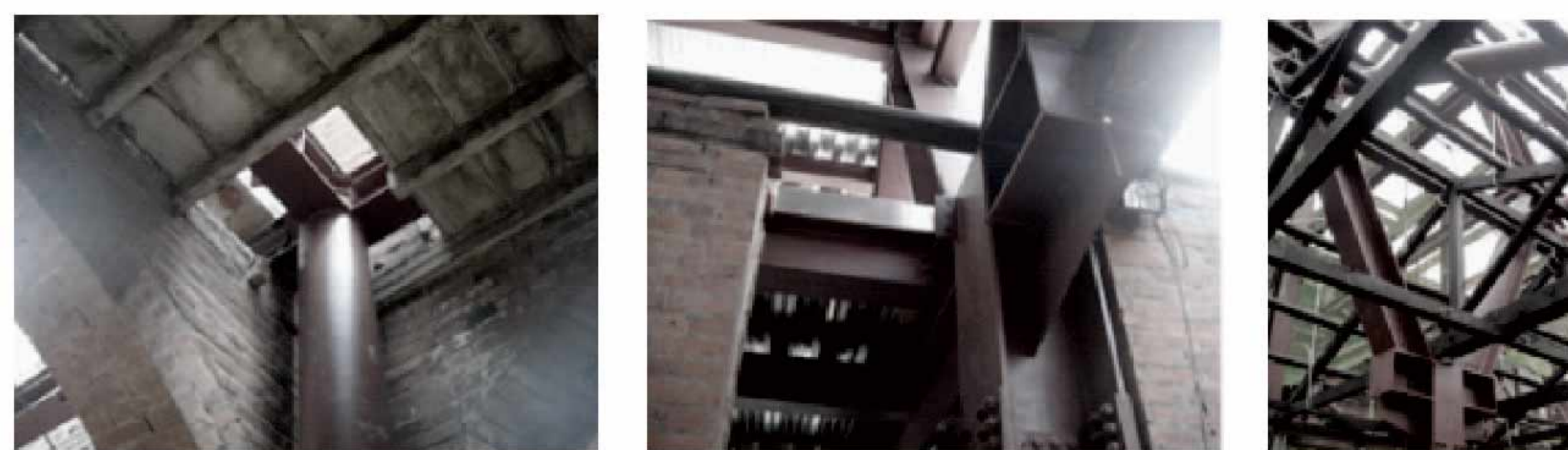
補強鋼構架與磚牆、磚柱、磚拱之關係
